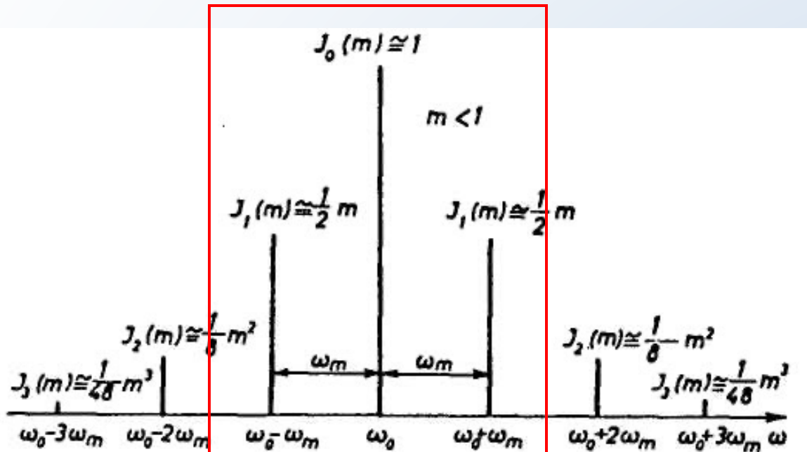
Slika: Dio amplitudskog spektra ugaono modulisanog signala sinusoidalnim test tonom sa indeksom modulacije m < 1
