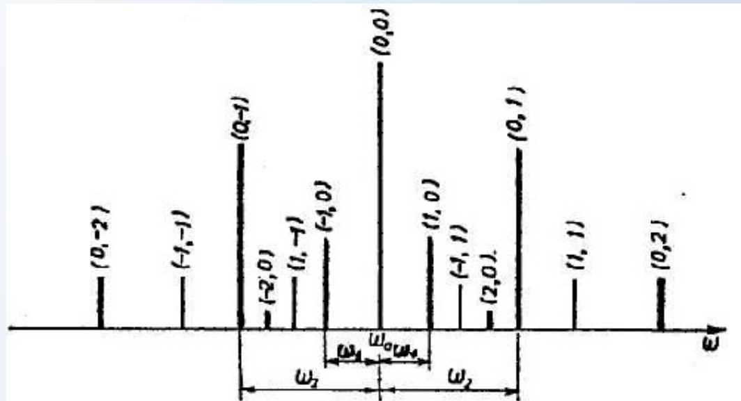
Slika: Amplitudski spektar ugaono modulisanog signala pri čemu je modulišućí signal sastavljen od sume dva sinusoidalna test tona čije su učestanosti \omega_1 i \omega_2 , a odgovarajućí indeksi modulacije m_1=0,5 i m_2=1
